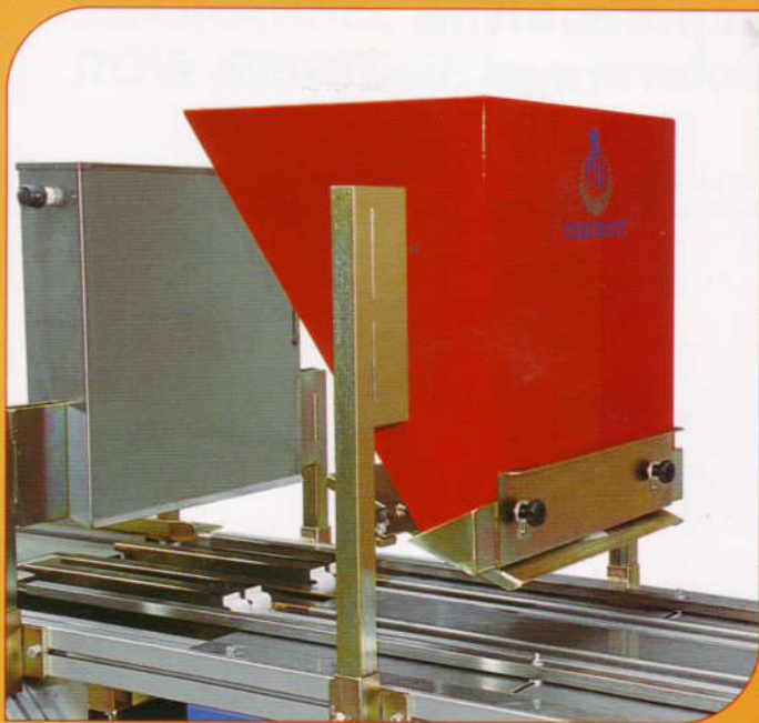
Particolare del copritore e bagnatore. A particular of the coverer and of the watering unit.
