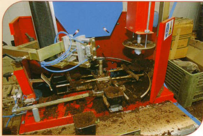
Particolare del distributore, del punzone rotante e dell'espulsore vasi. A particular of the pot denester, of the drilling unit of the pot take off arm.
